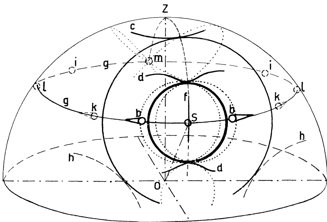
FIG. 2. — Aspects principaux des phénomènes de halo : o : observateur — s : soleil au centre du halo principal de 22^\circ et du grand halo de 46^\circ — b : parhémie de 22^\circ (environ) — c : arc circumzénital tangent au grand halo — d : arcs tangents supérieur et inférieur — f : colonne lumineuse et croix — g : cercle parhélique — h : arcs tangents infralatéraux — i : parhélies de 120^\circ — k : parhélies de 46^\circ (environ) — l : parhélies de 90^\circ — m : anthémie.
